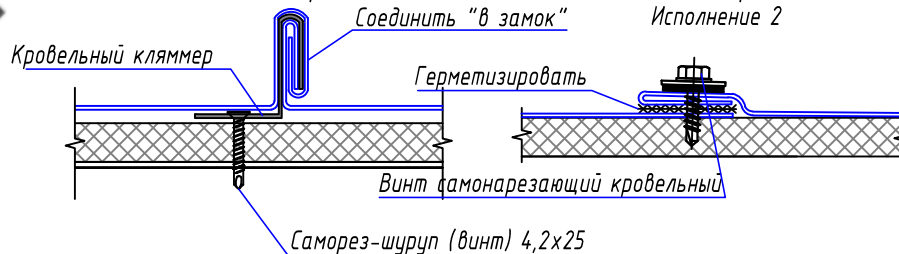
Узел стыковки стальных листов покрытия на парапете Исполнение 1: с двойным фальцем (возможно исполнение с лежащем фальцем) Соединить "в замок" Исполнение 2
